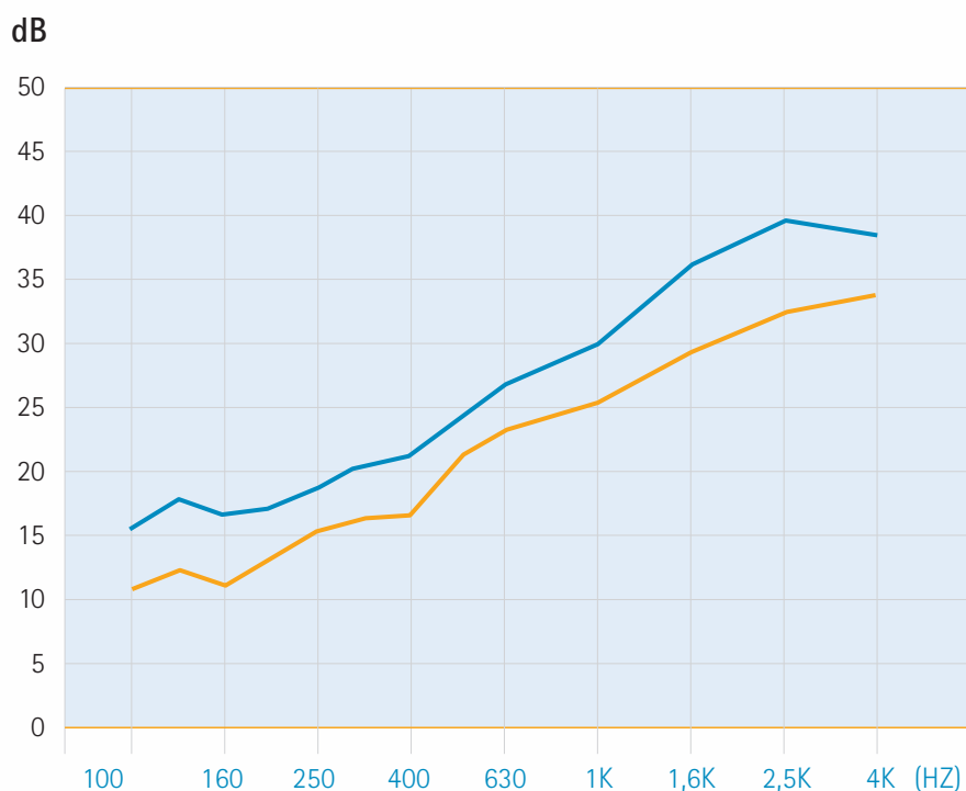
GRÁFICO DE AISLAMIENTO ACÚSTICO QUE PROPORCIONA EL METAMAD
